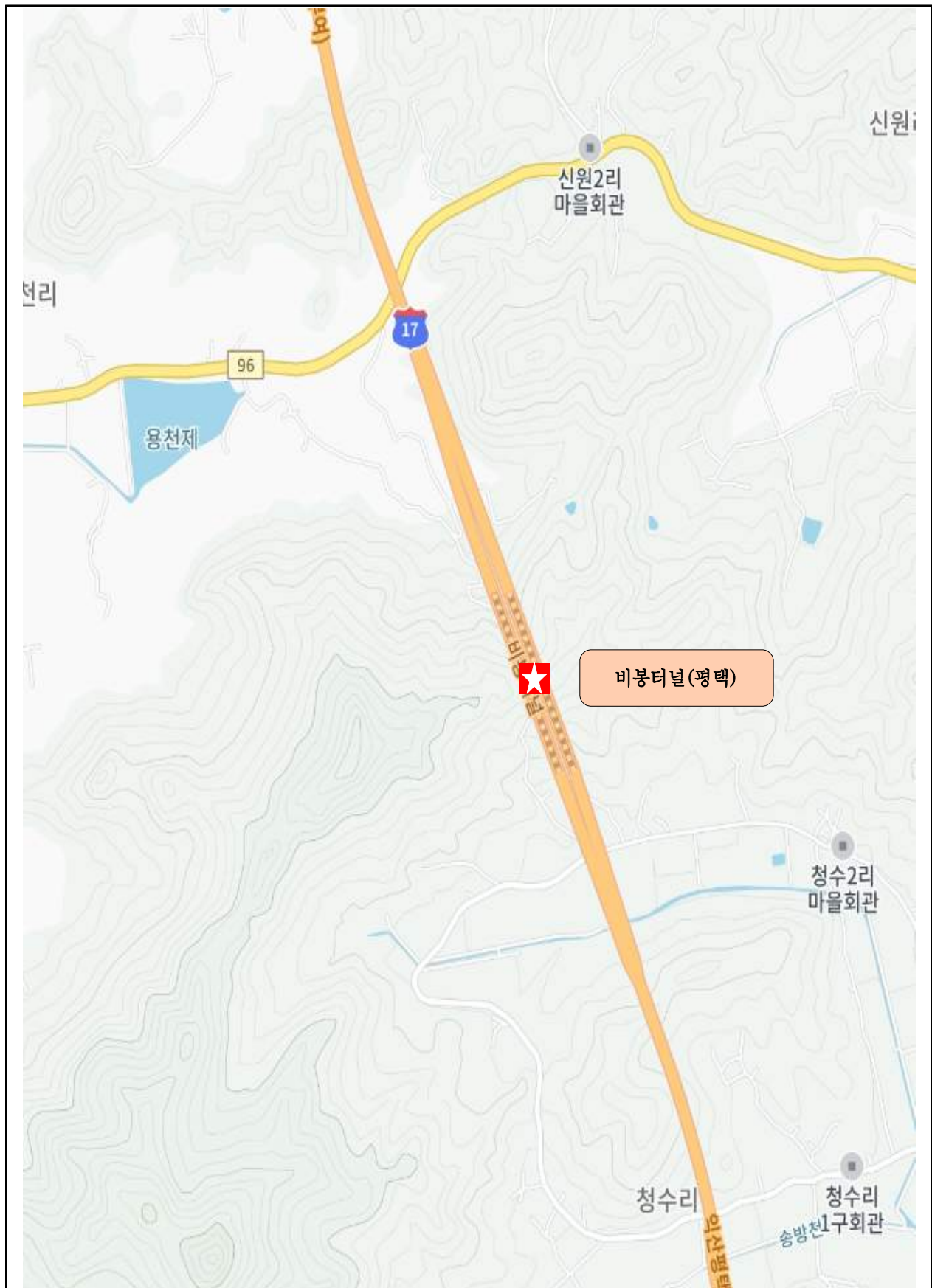
【그림 2.10.1】 위치도
